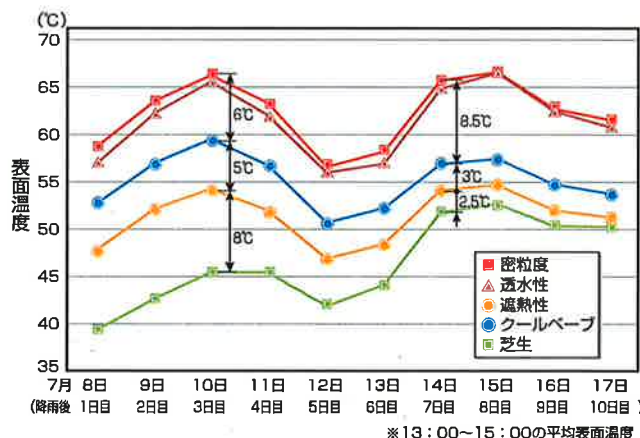
【図2】 舗装材による表面温度形成
