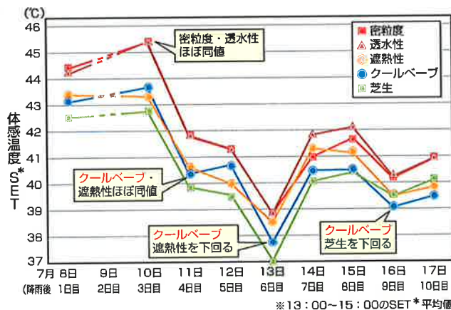
【図5】 各舗装材上の体感温度SET*の経時変動
