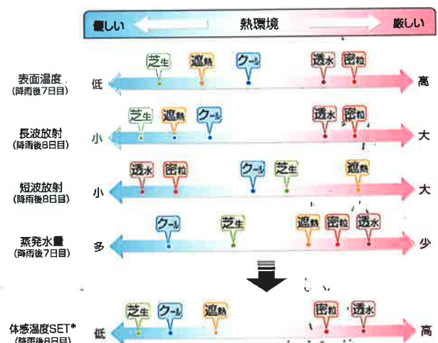
【図6】 各舗装材の熱的条件別の性能比較
